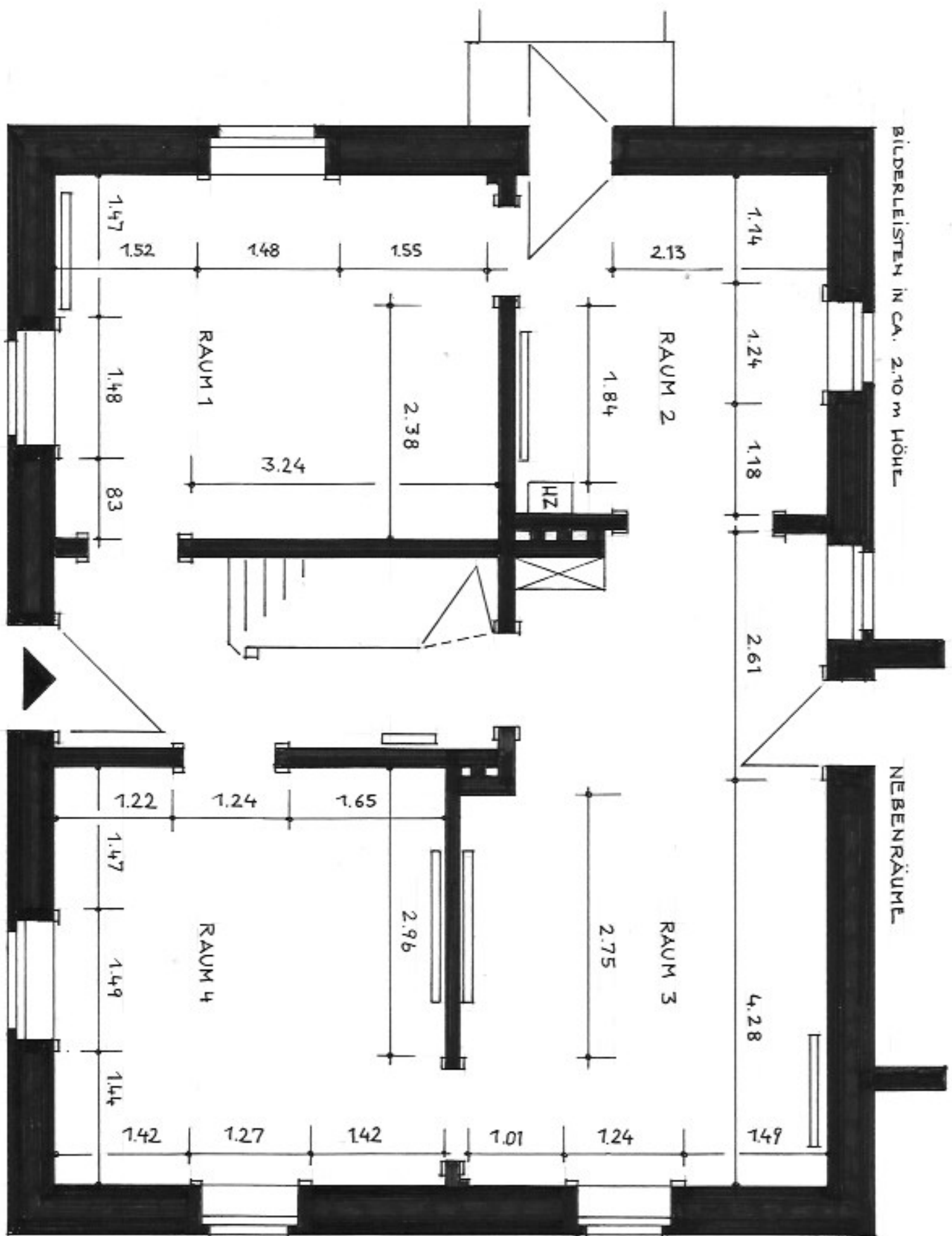
HÄNGEPLAN SCHLEUSENH AUS
